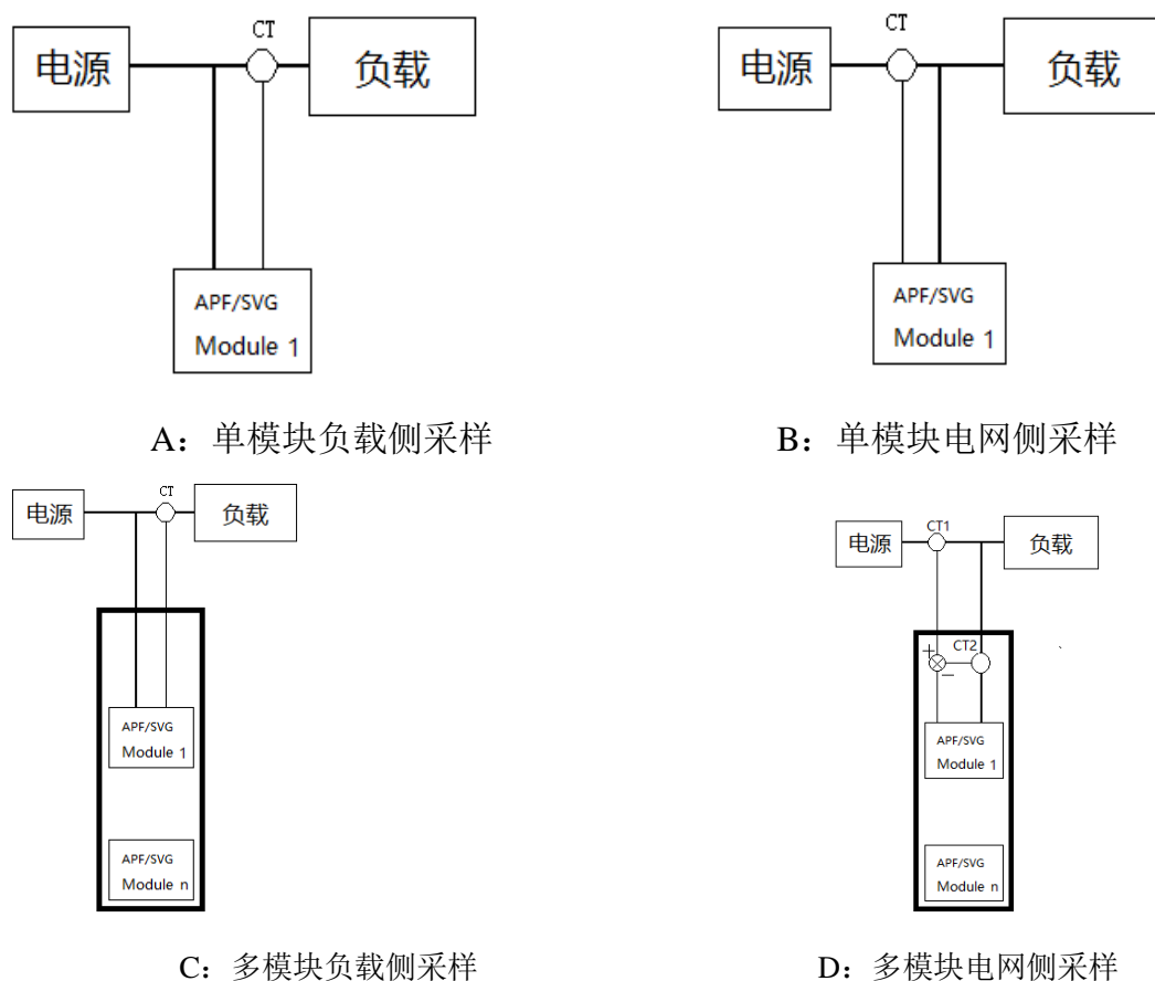
图 4-5 安装示意图
