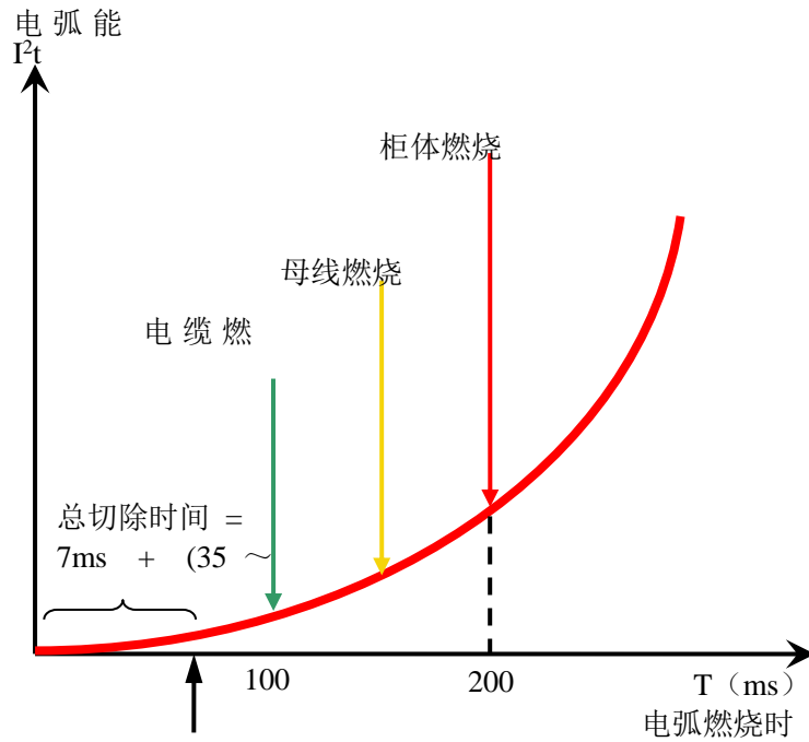
电弧光危害示意
